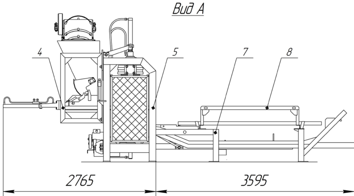
Рисунок 1. Общая компоновка комплекса (продолжение).
