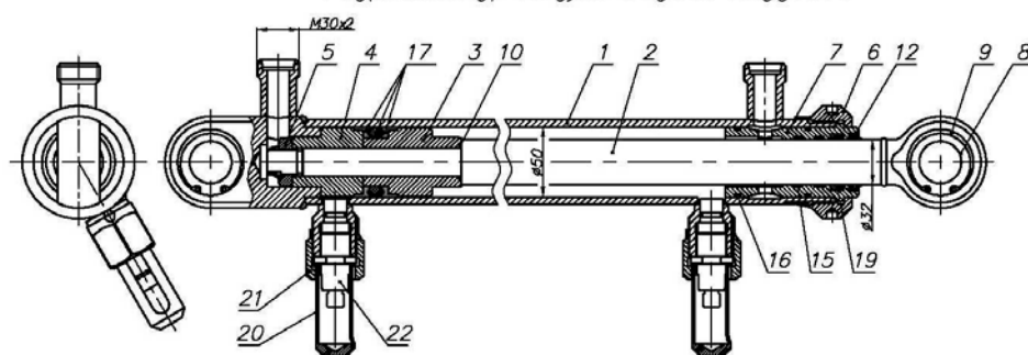
Гидроцилиндр модуля подачи поддонов
