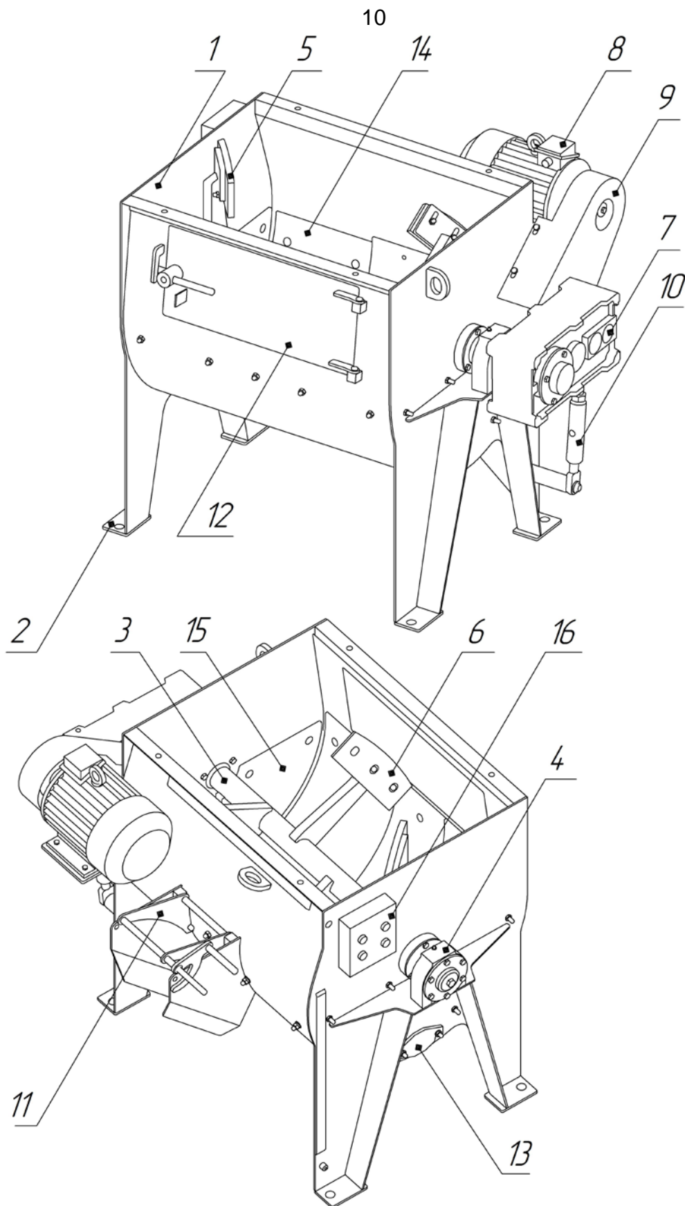
Рисунок 4. Смеситель
