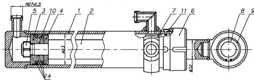
Гидроцилиндр матрицы
