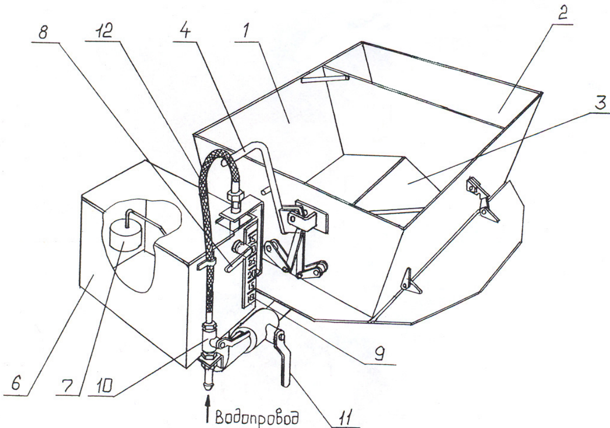
Рисунок 3. Дозатор компонентов смеси
