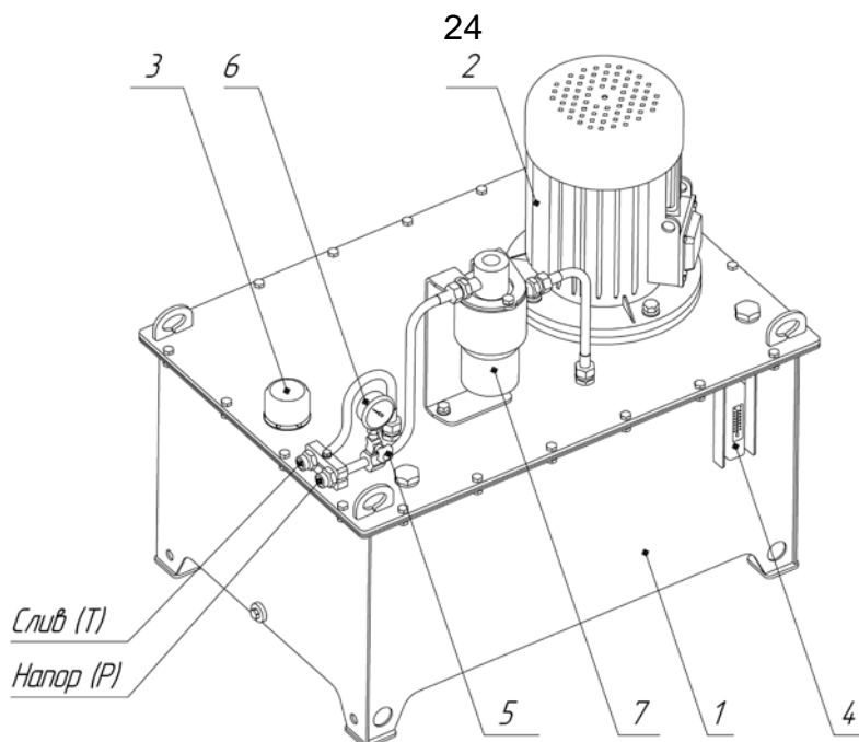
Рисунок 18 – Установка насосная
