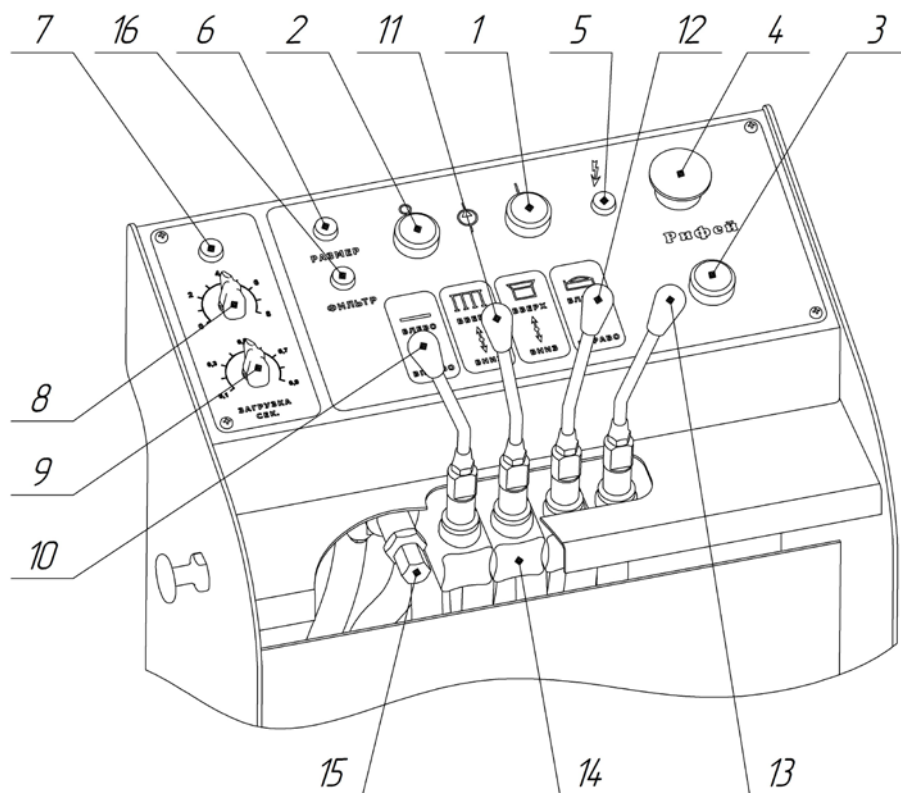
Рисунок 15. Панель управления.
