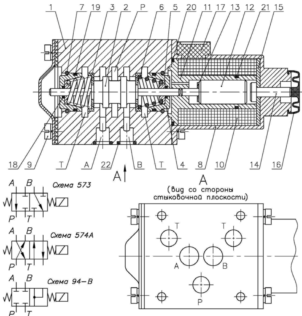
Рисунок 20. Устройство и принцип работы гидрораспределителя
