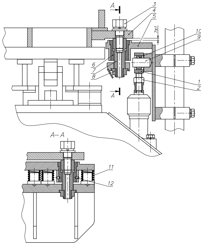
Рисунок 27. Схема настройки прижима матрицы.
