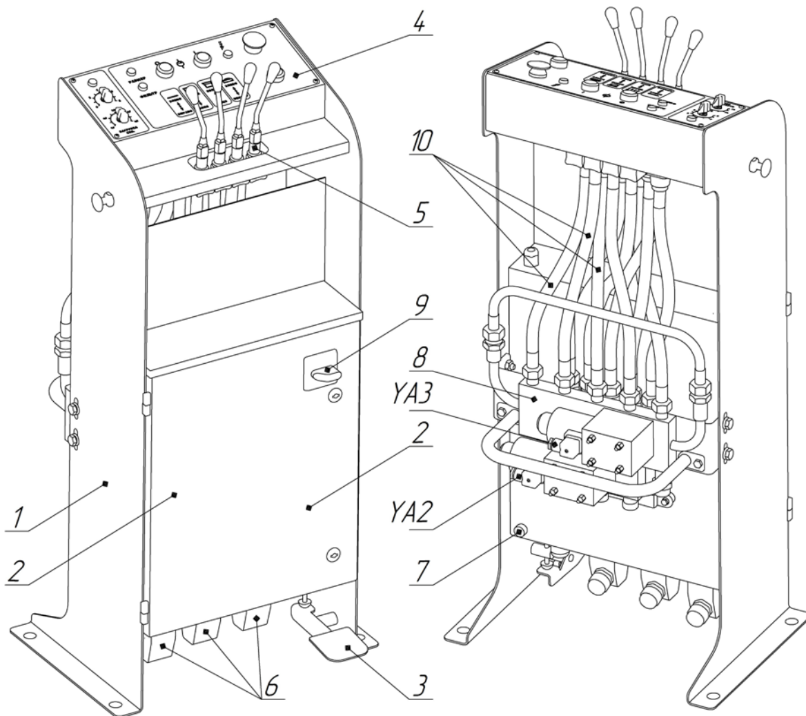
Рисунок 14. Пульт управления.
