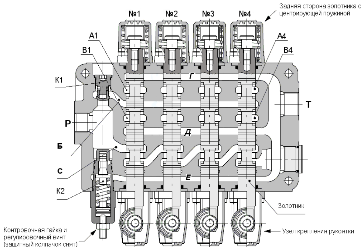
Рисунок 21. Гидрораспределитель ручной HC-D10/4-IR201 (110)
