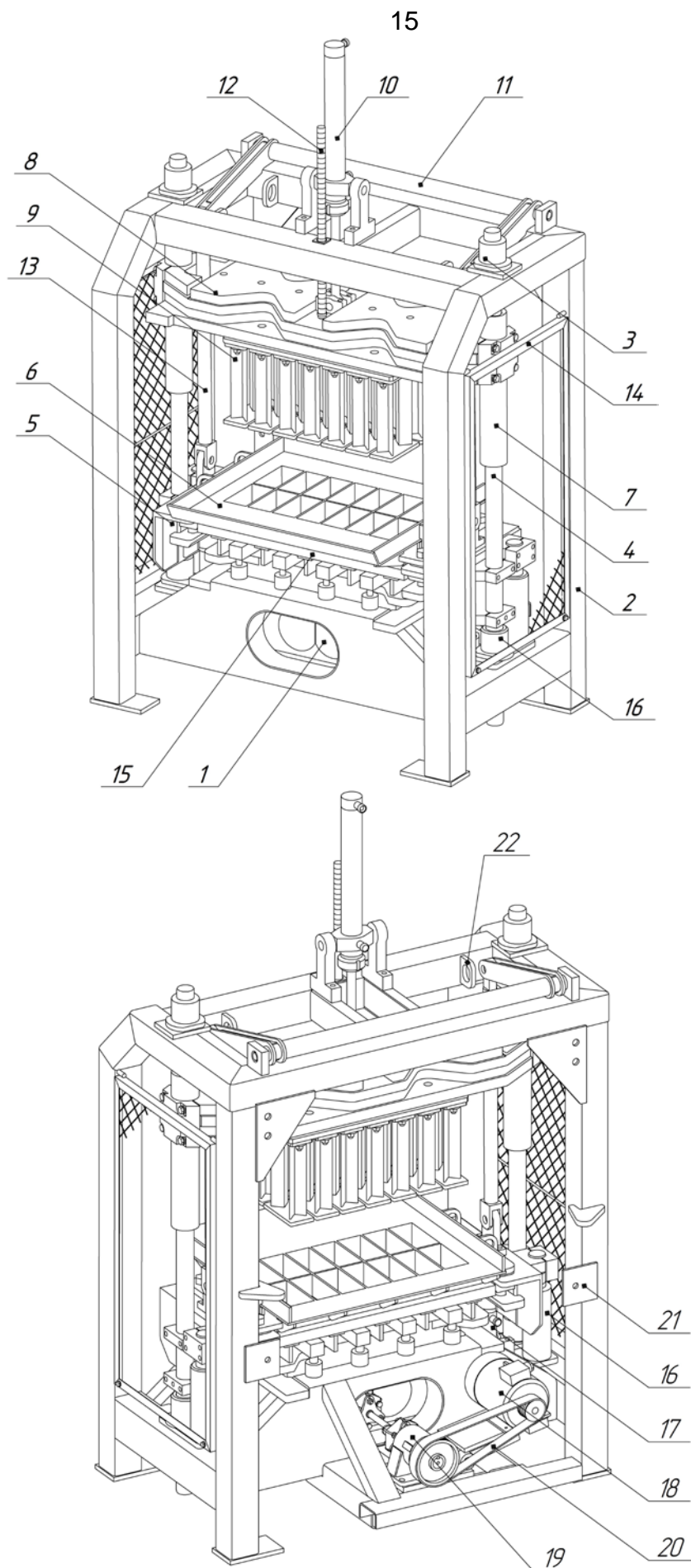
Рисунок 9. Вибропресс .
