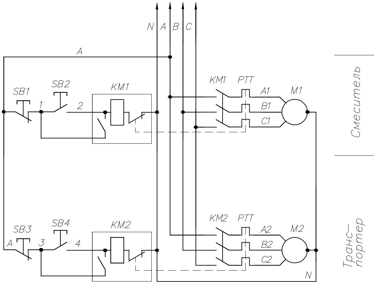
Рисунок 23. Схема электрическая принципиальная смесителя.
