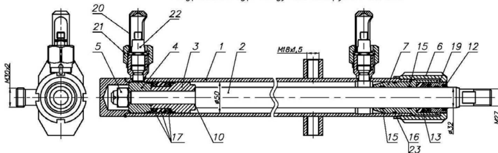
Гидроцилиндр модуля подачи поддонов
