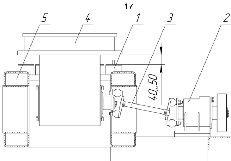
Рисунок 11. Проверка подушек вибростола.
