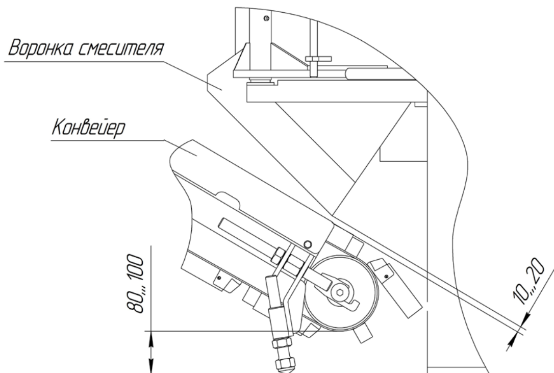
Рисунок 7. Настройка зазора между смесителем и транспортером.
