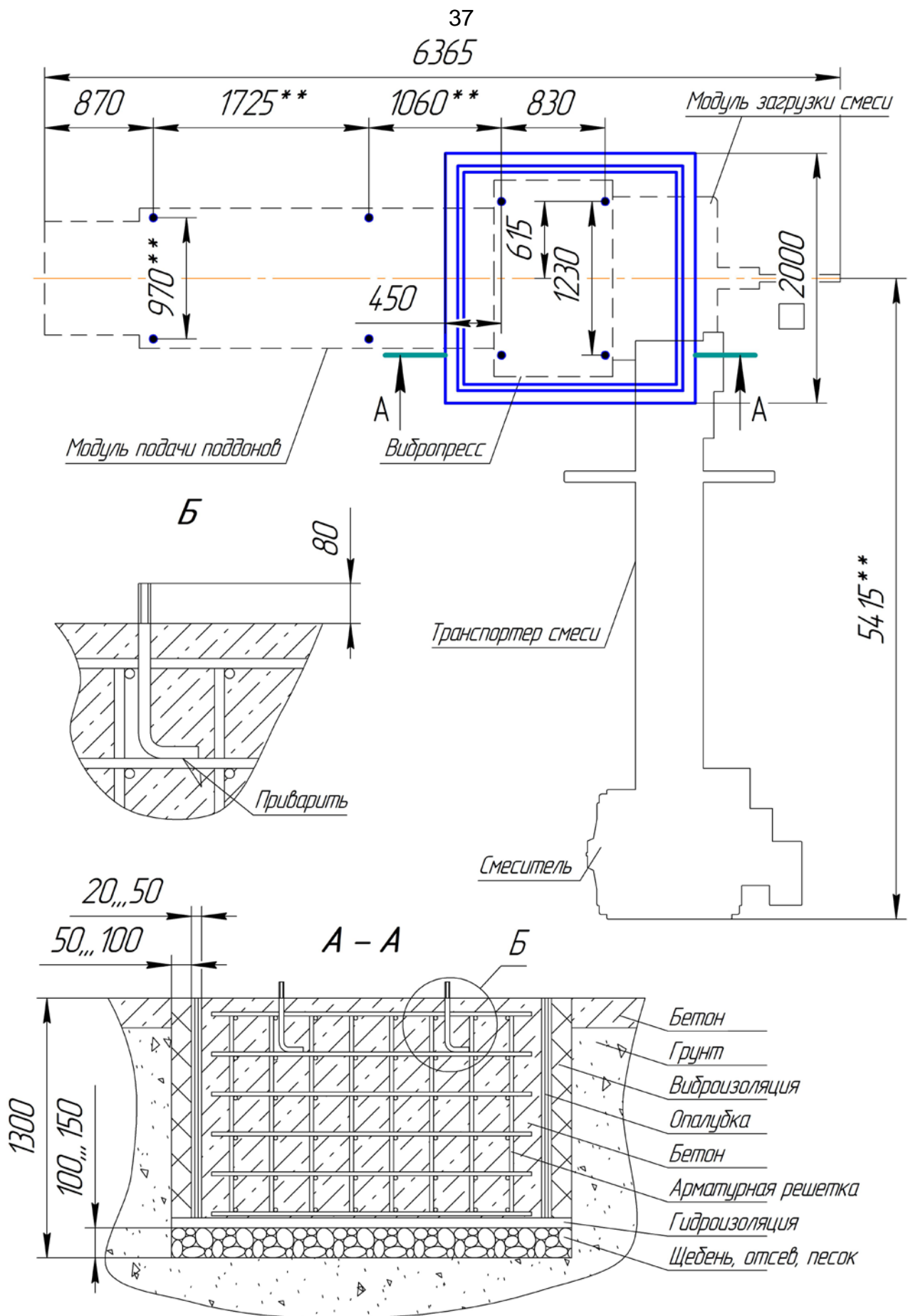
Рисунок 26. Схема фундамента комплекса.
