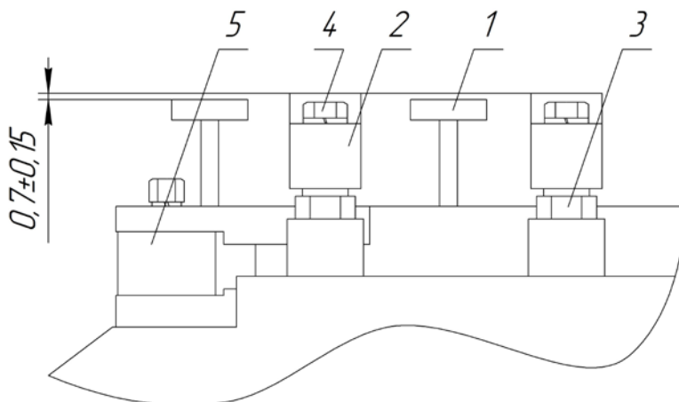
Рисунок 10. Настройка вибростола.
