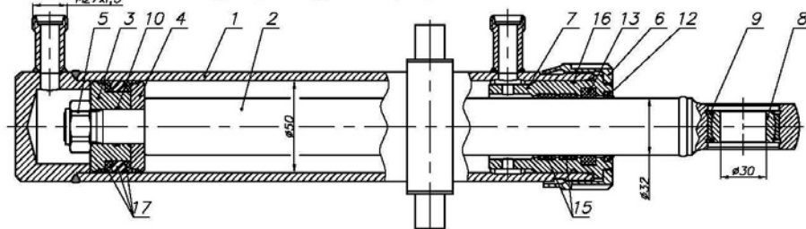
Гидроцилиндр модулей загрузки смеси
