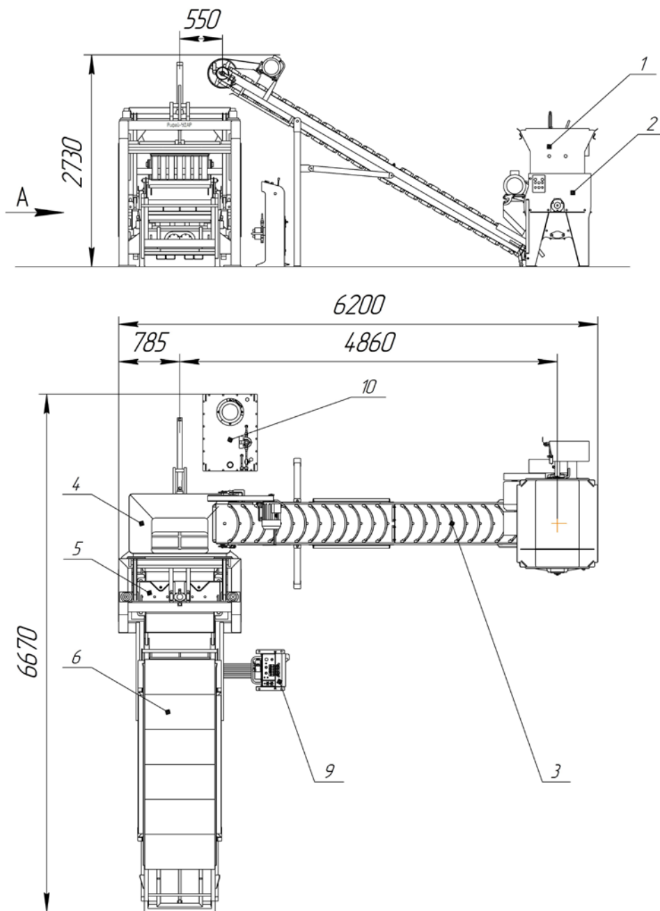
Рисунок 1. Общая компоновка комплекса.
