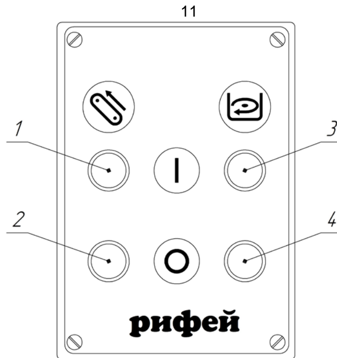
Рис. 5. Пульт управления смесителем и транспортером 1 - включение транспортера смеси; 2 - отключение транспортера смеси; 3 - включение смесителя; 4 - отключение смесителя.
