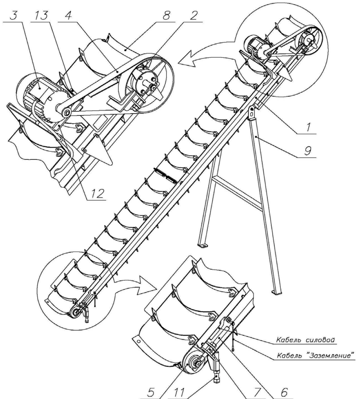
Рисунок 6. Конвейер смеси.
