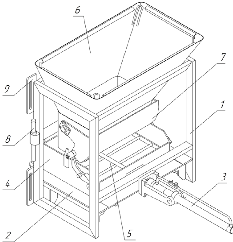
Рисунок 12. Модуль загрузки смеси.
